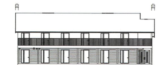
北立面図
